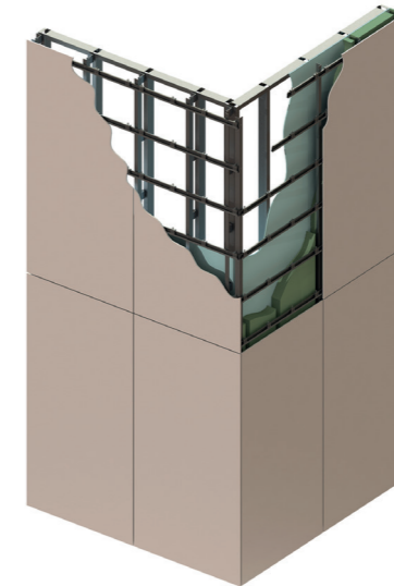
Cassette-Fix Assembly
