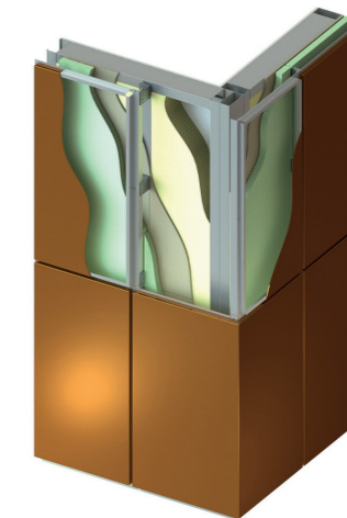
Cassette-Fix Assembly
